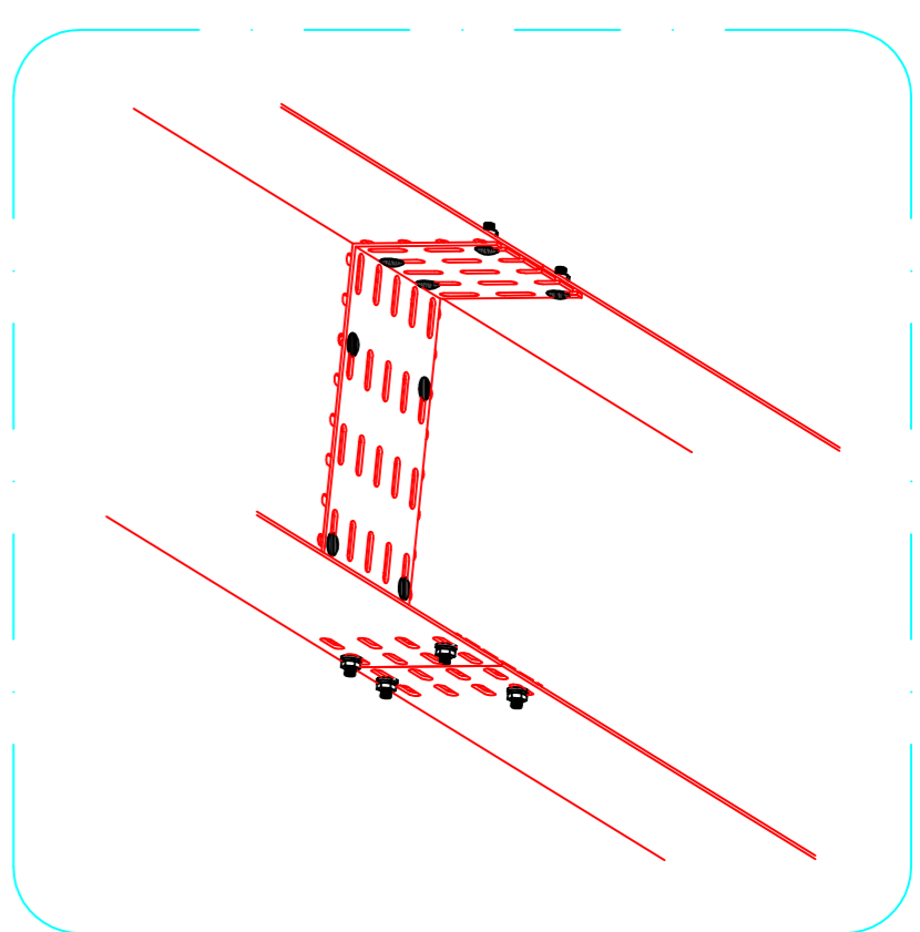
DETALHE FIXAÇÃO JUNÇÃO DE ELETRICALHA
