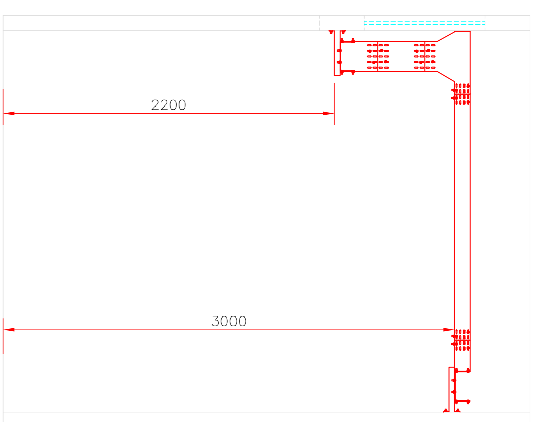
CORTE B-B - DETALHE ALTURA FIXAÇÃO ELETROCALHA ESC. 1:25
